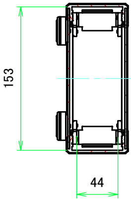
A-A ( 1:4 )
