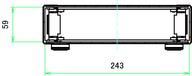
B-B ( 1:4 )
